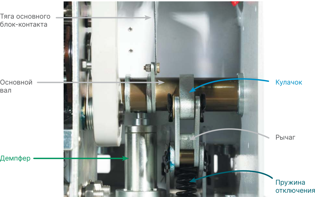
РИСУНОК 8. МЕХАНИЗМ ОТКЛЮЧЕНИЯ
