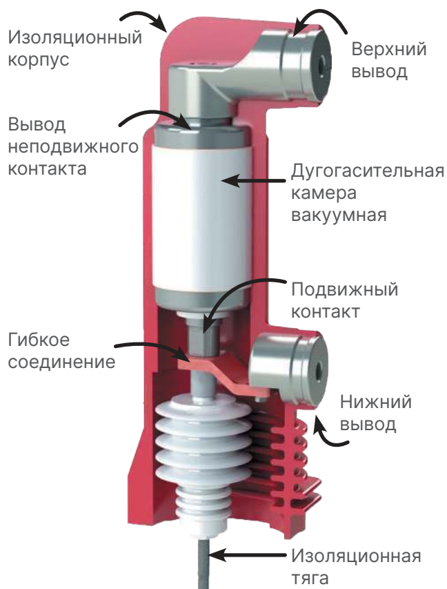
РИСУНОК 1. ПОЛЮС ВЫКЛЮЧАТЕЛЯ
