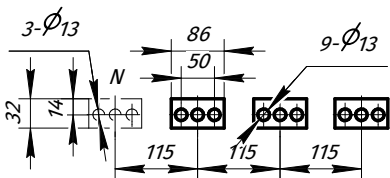
Шинные выводы
